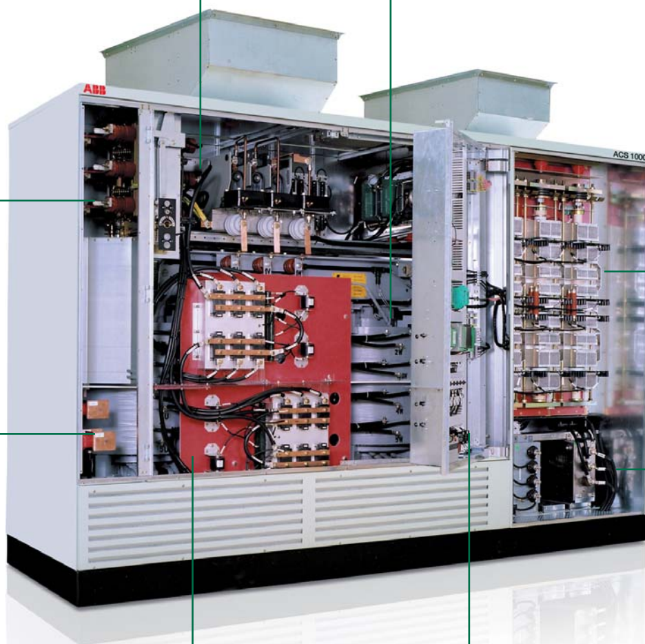
24-пульсный входной выпрямитель в стандартном исполнении
